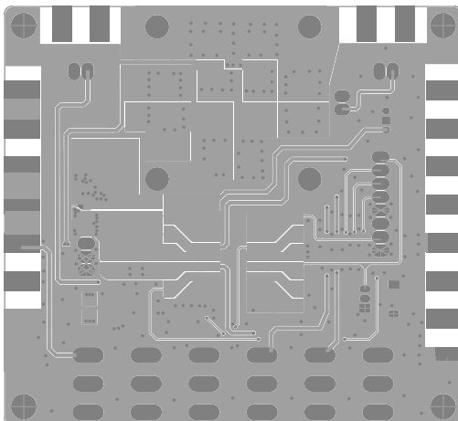
图 6、底层镜像
