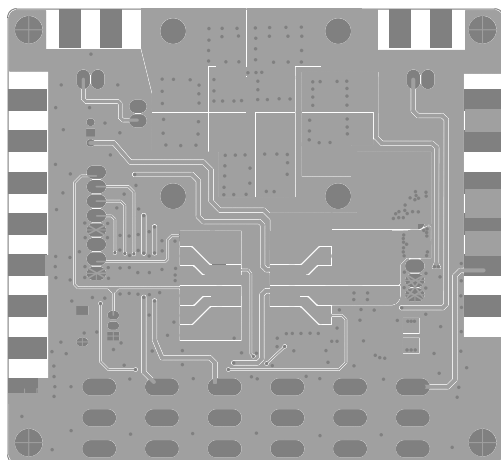
图 5、底层
