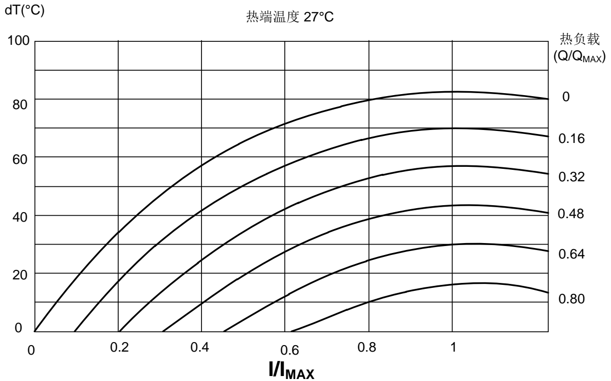
图 13. dT vs. I/Imax
