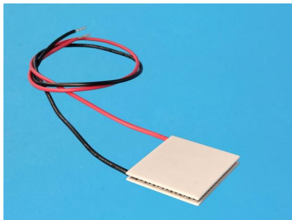
图 2. ATE1-TCHE-71 的立体照片
