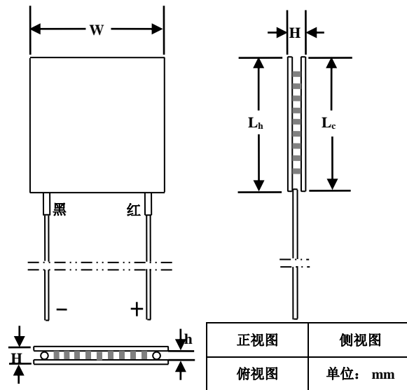
图21. 非密封ATE1-TCHE-71的机械尺寸
