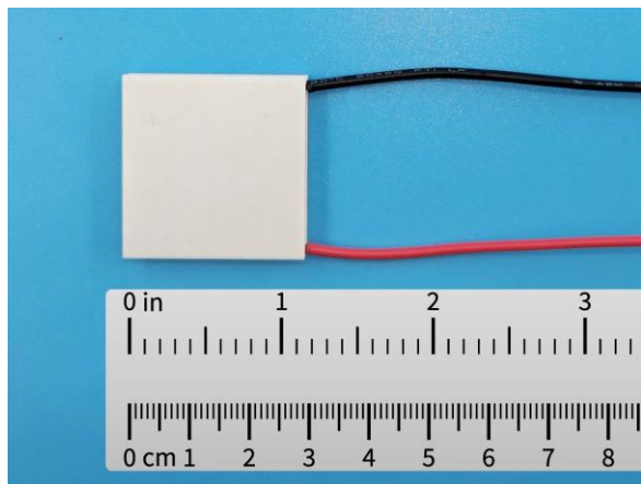
图 1. TE1-TCHE-71 的照片
