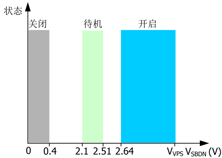
图 3、 V_{SBDN} VS. 放大器状态
